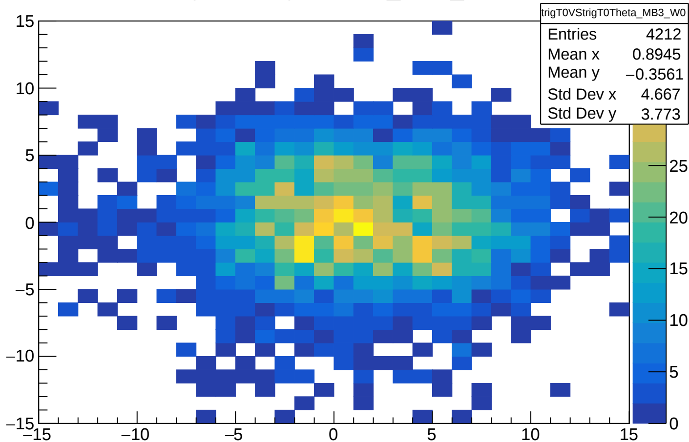
trigT0VStrigT0Theta_MB3_W0
