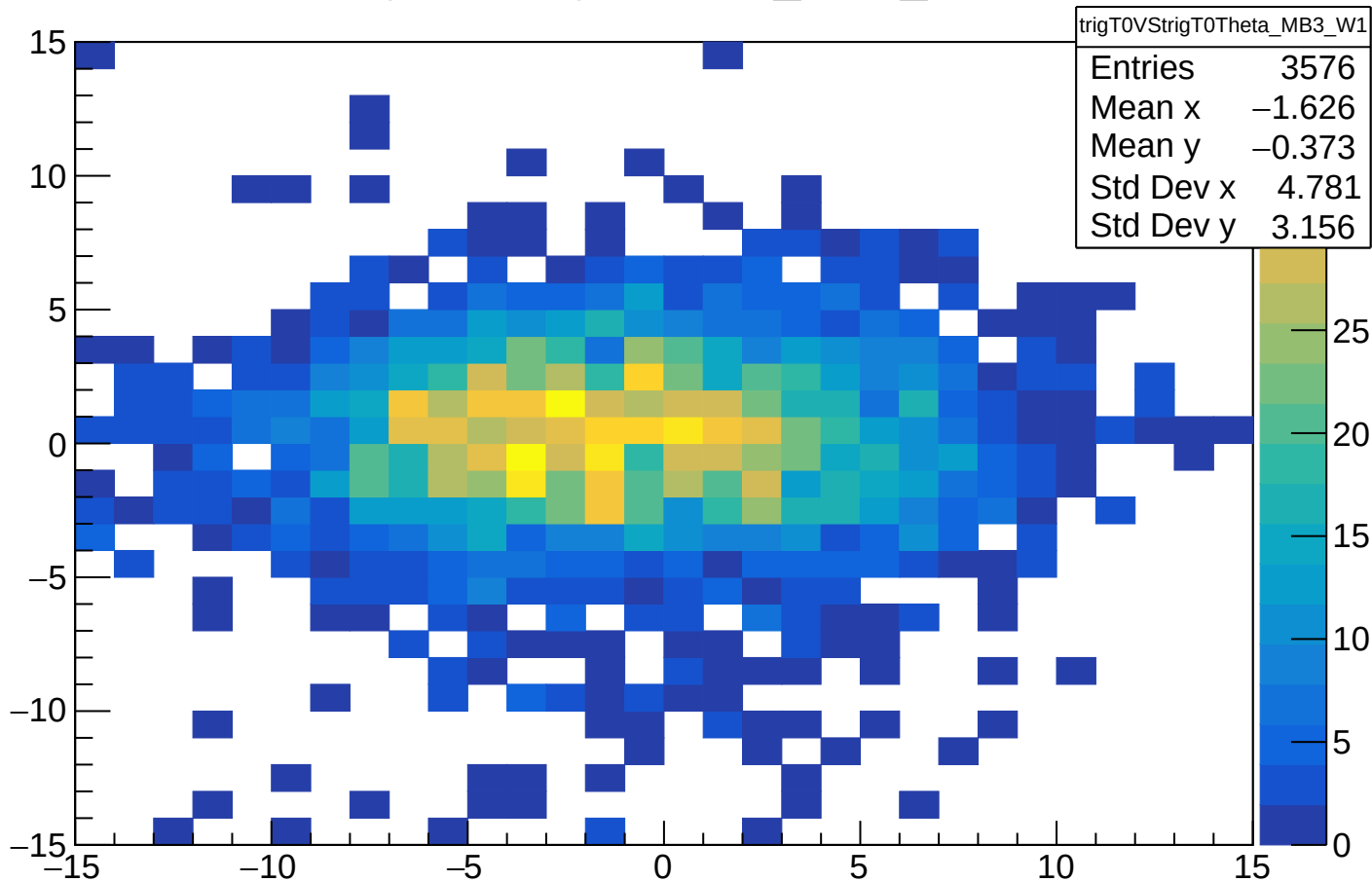
trigT0VStrigT0Theta_MB3_W1
