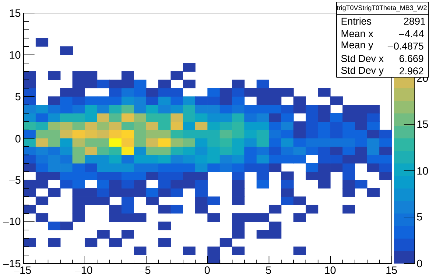
trigT0VStrigT0Theta_MB3_W2
