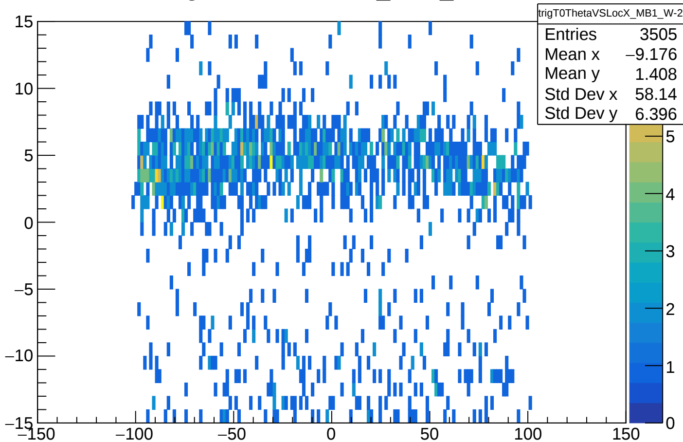
trigT0ThetaVSLocX_MB1_W-2
