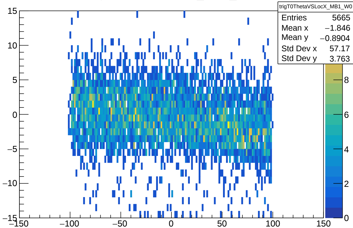
trigT0ThetaVSLocX_MB1_W0
