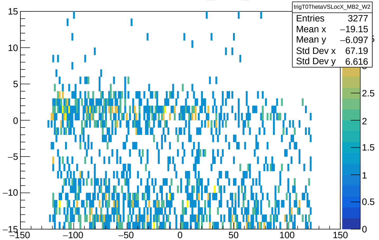
trigT0ThetaVSLocX_MB2_W2
