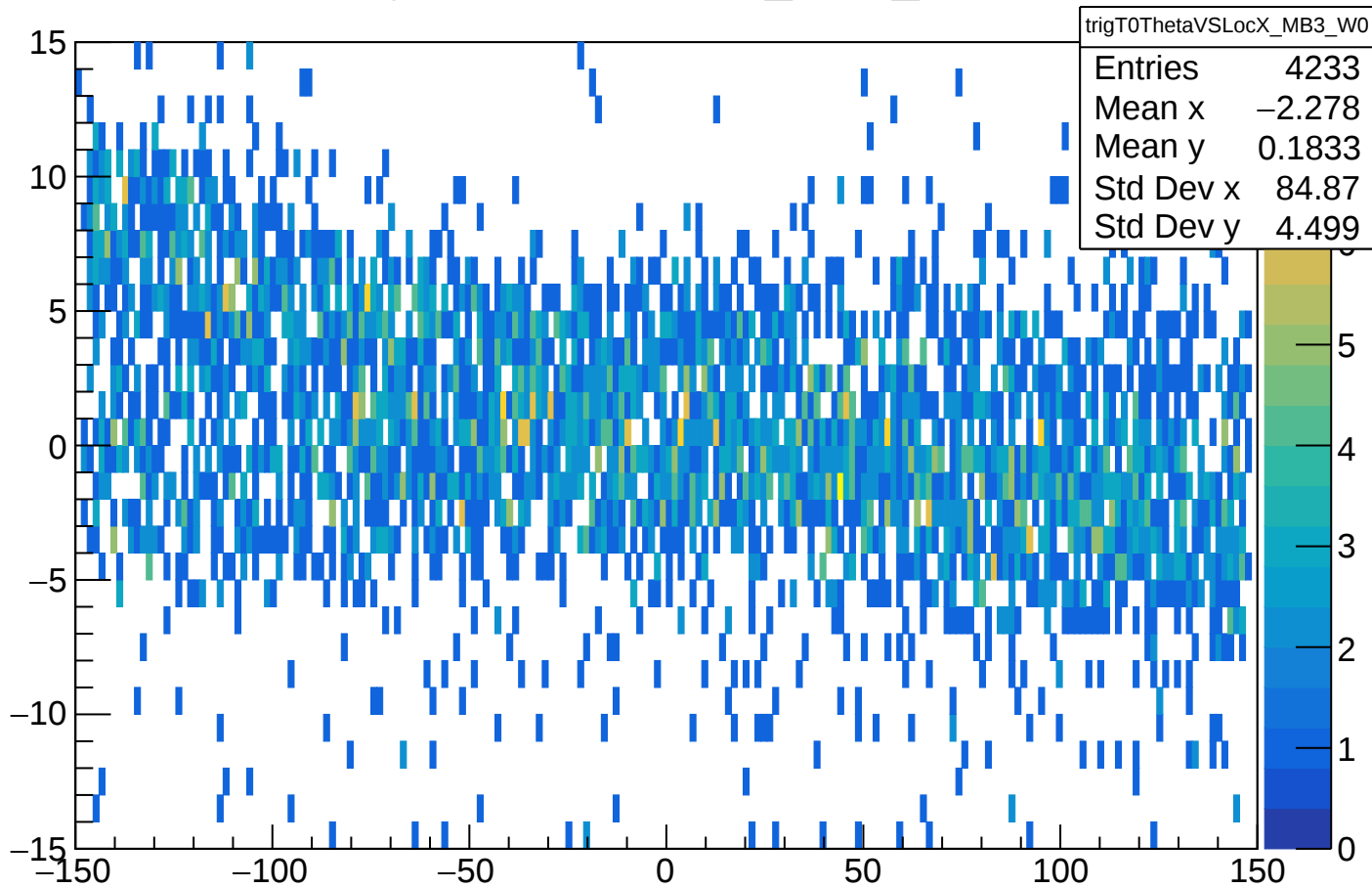
trigT0ThetaVSLocX_MB3_W0
