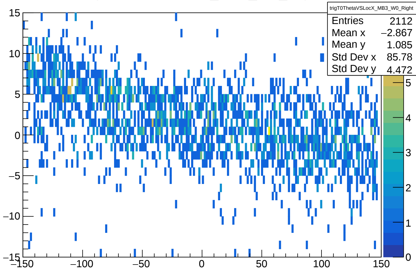
trigT0ThetaVSLocX_MB3_W0_Right
