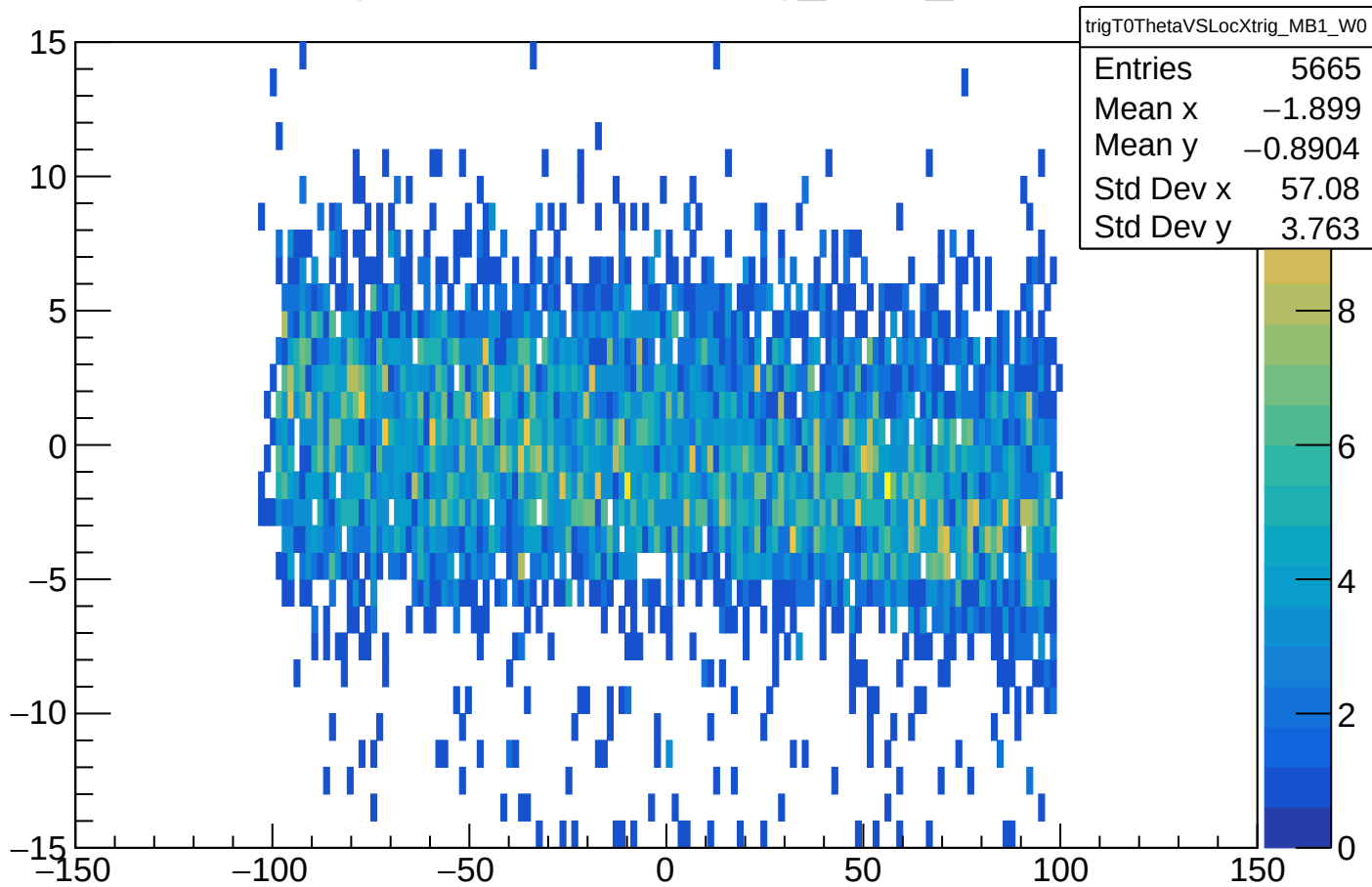
trigT0ThetaVSLocXtrig_MB1_W0
