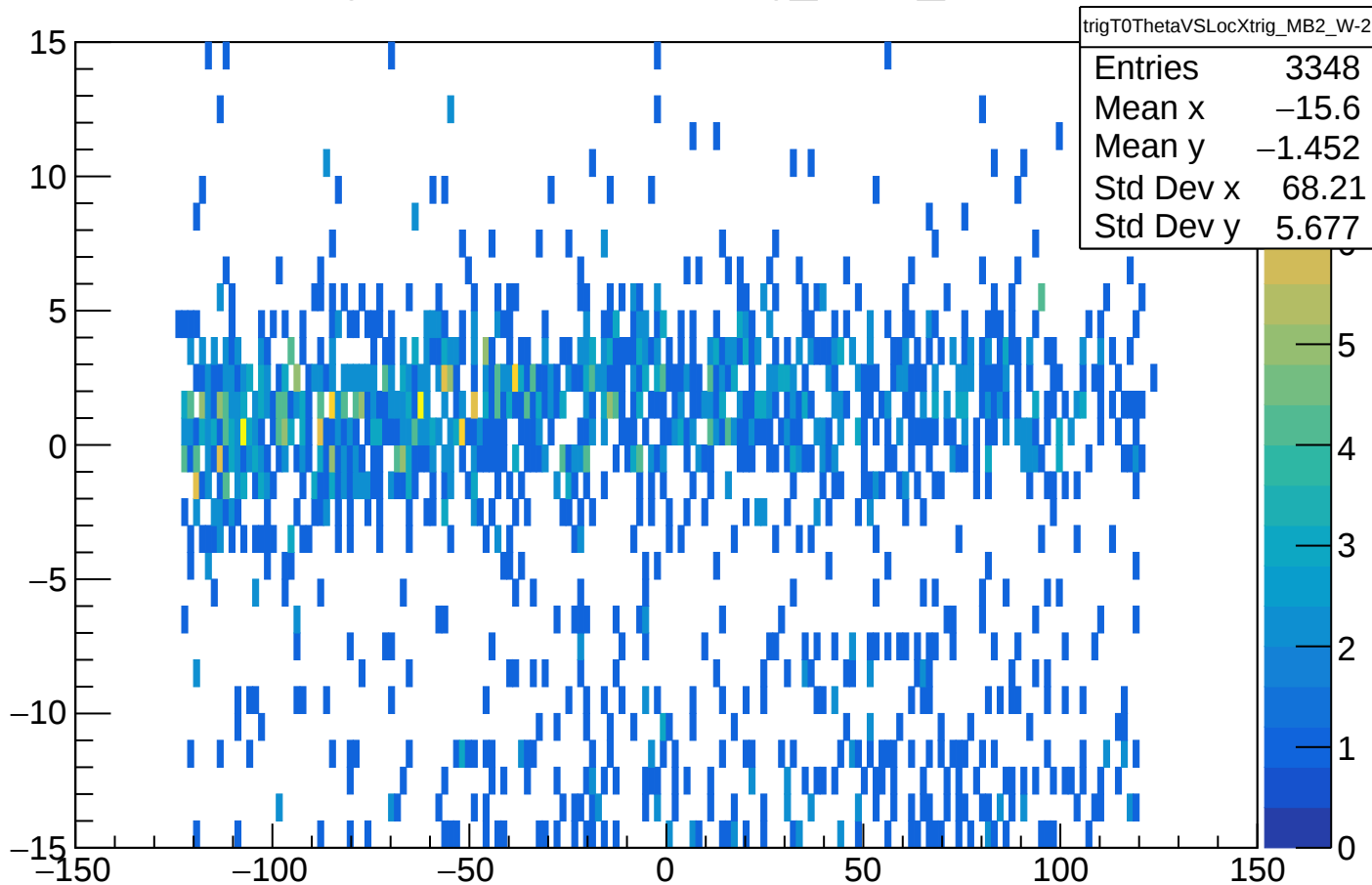
trigT0ThetaVSLocXtrig_MB2_W-2
