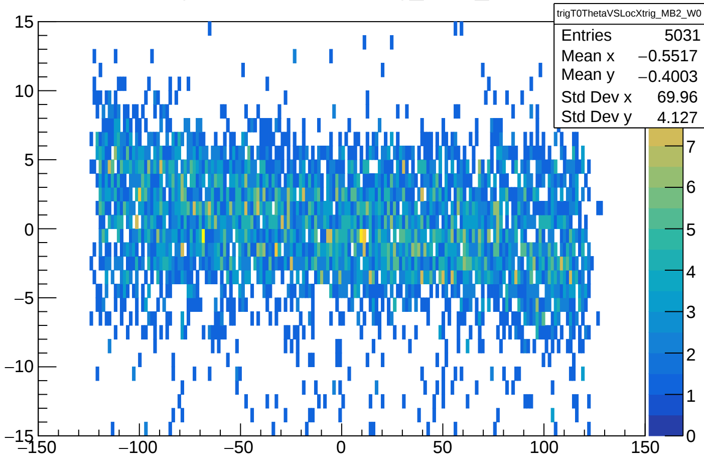
trigT0ThetaVSLocXtrig_MB2_W0
