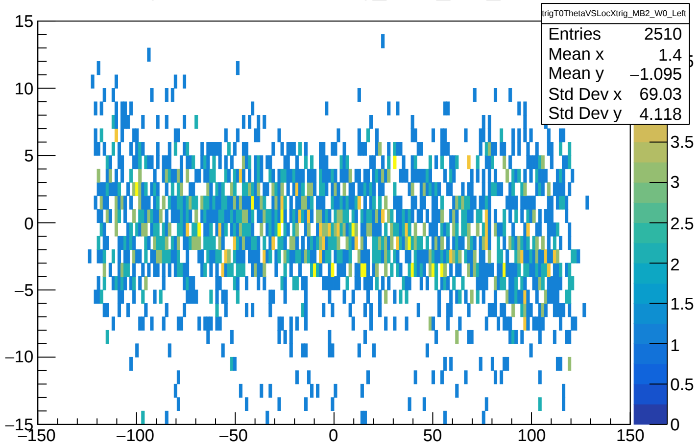
trigT0ThetaVSLocXtrig_MB2_W0_Left
