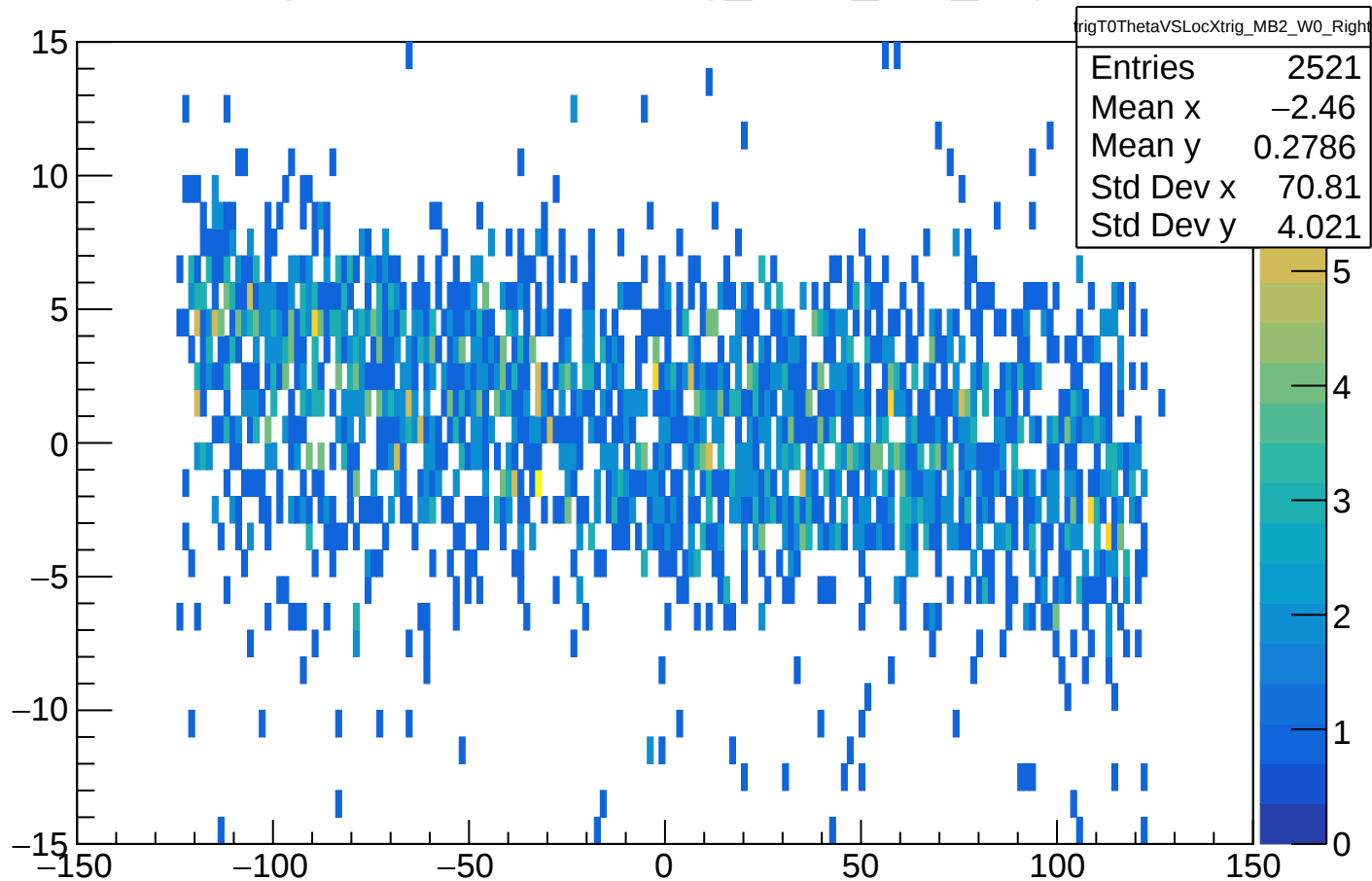
trigT0ThetaVSLocXtrig_MB2_W0_Right
