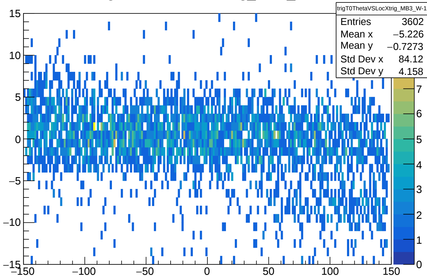
trigT0ThetaVSLocXtrig_MB3_W-1
