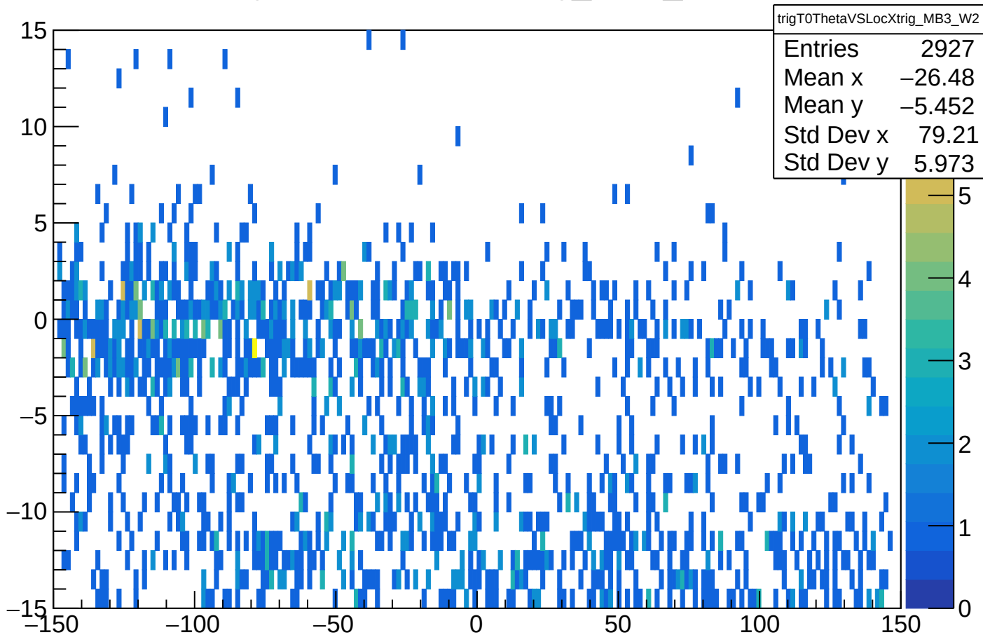
trigT0ThetaVSLocXtrig_MB3_W2
