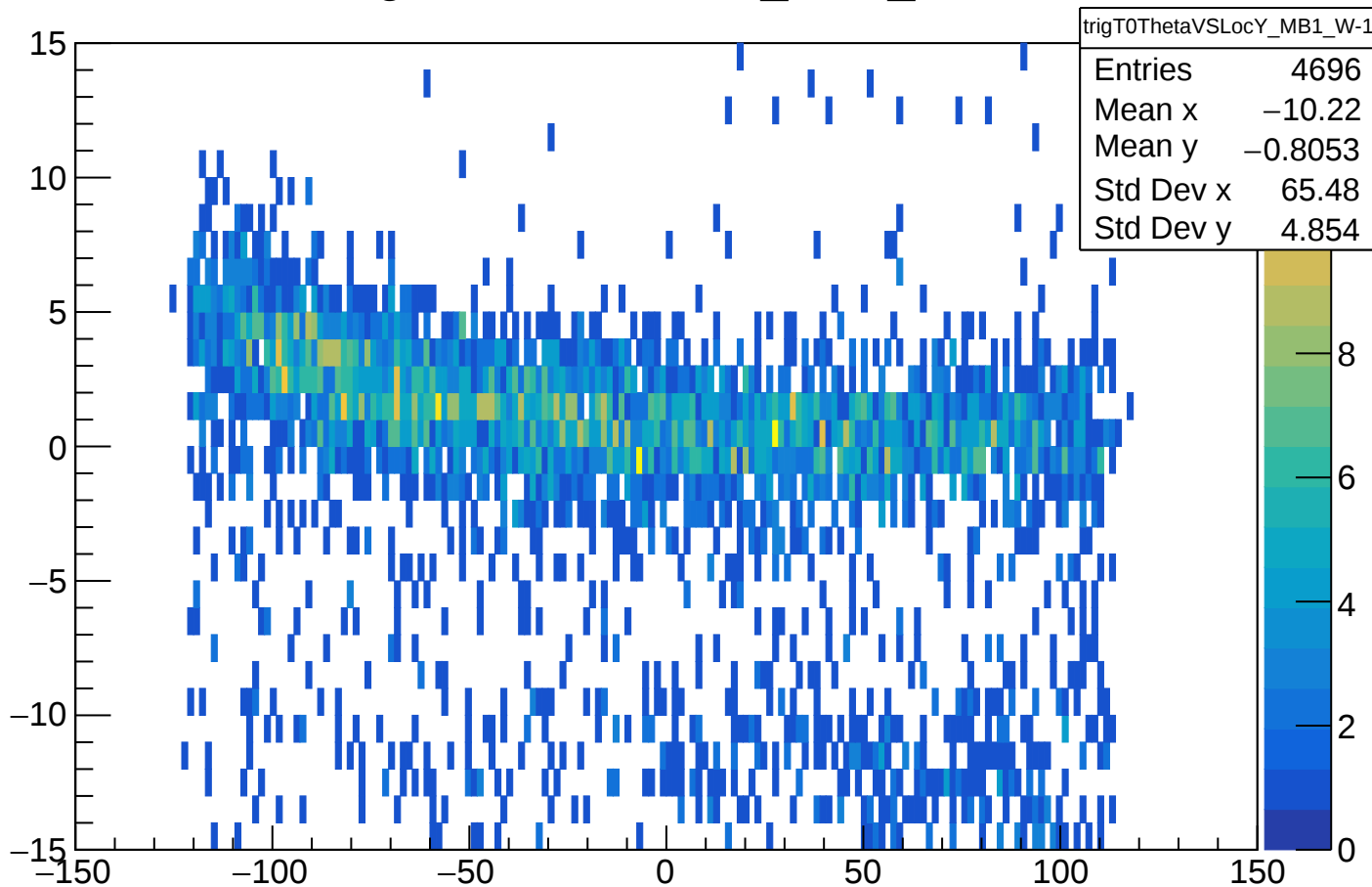
trigT0ThetaVSLocY_MB1_W-1
