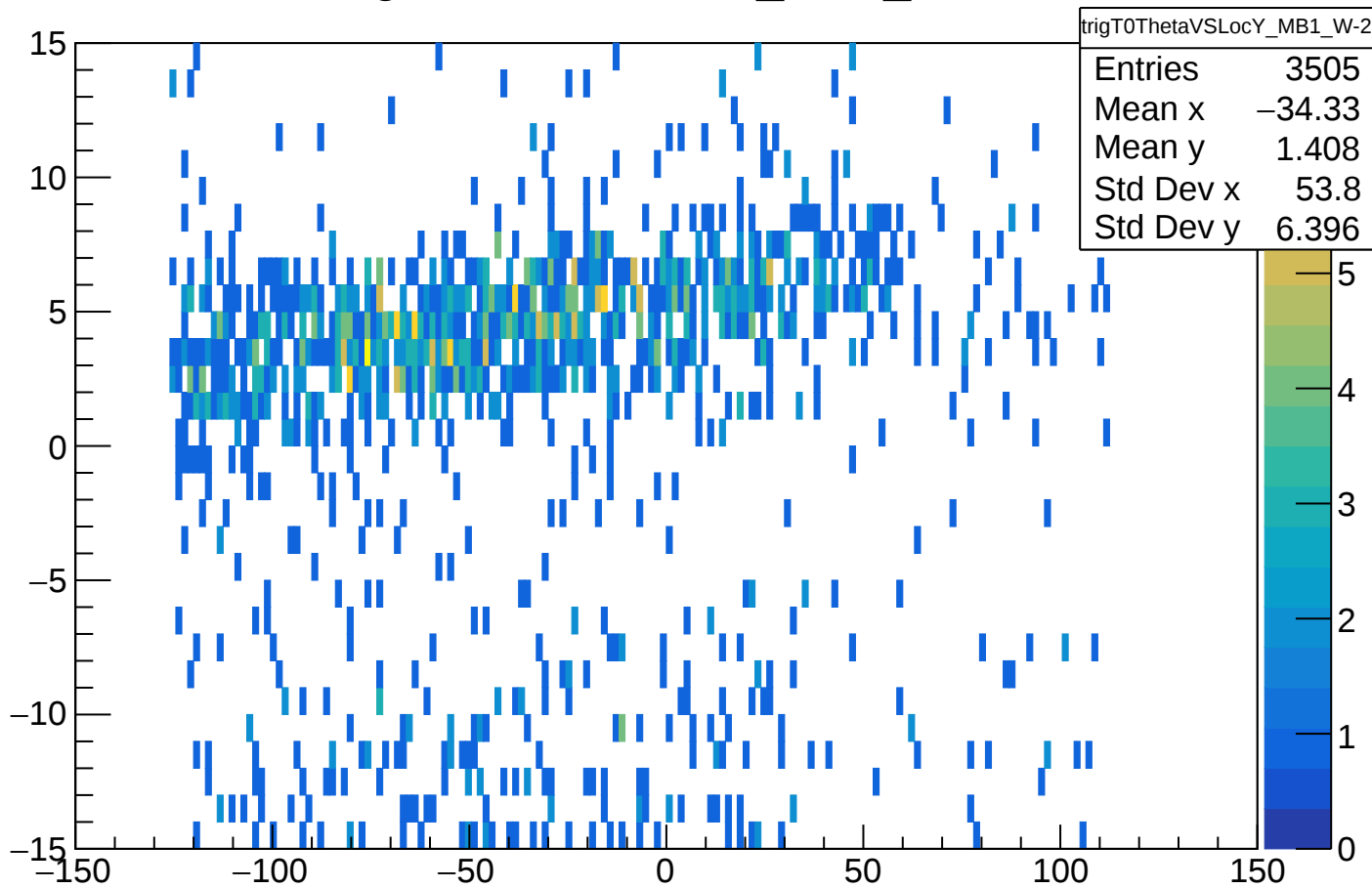
trigT0ThetaVSLocY_MB1_W-2
