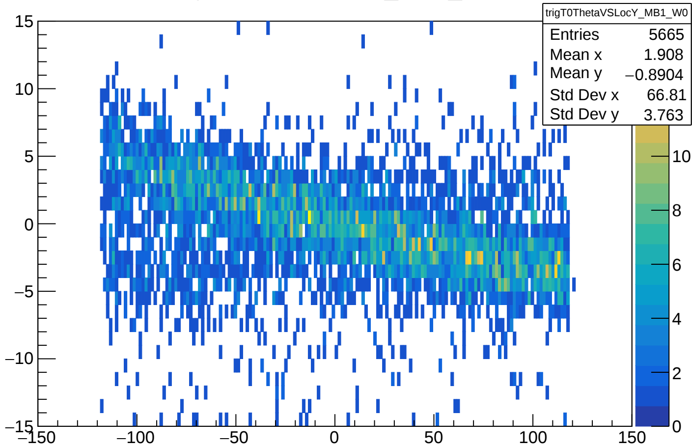
trigT0ThetaVSLocY_MB1_W0
