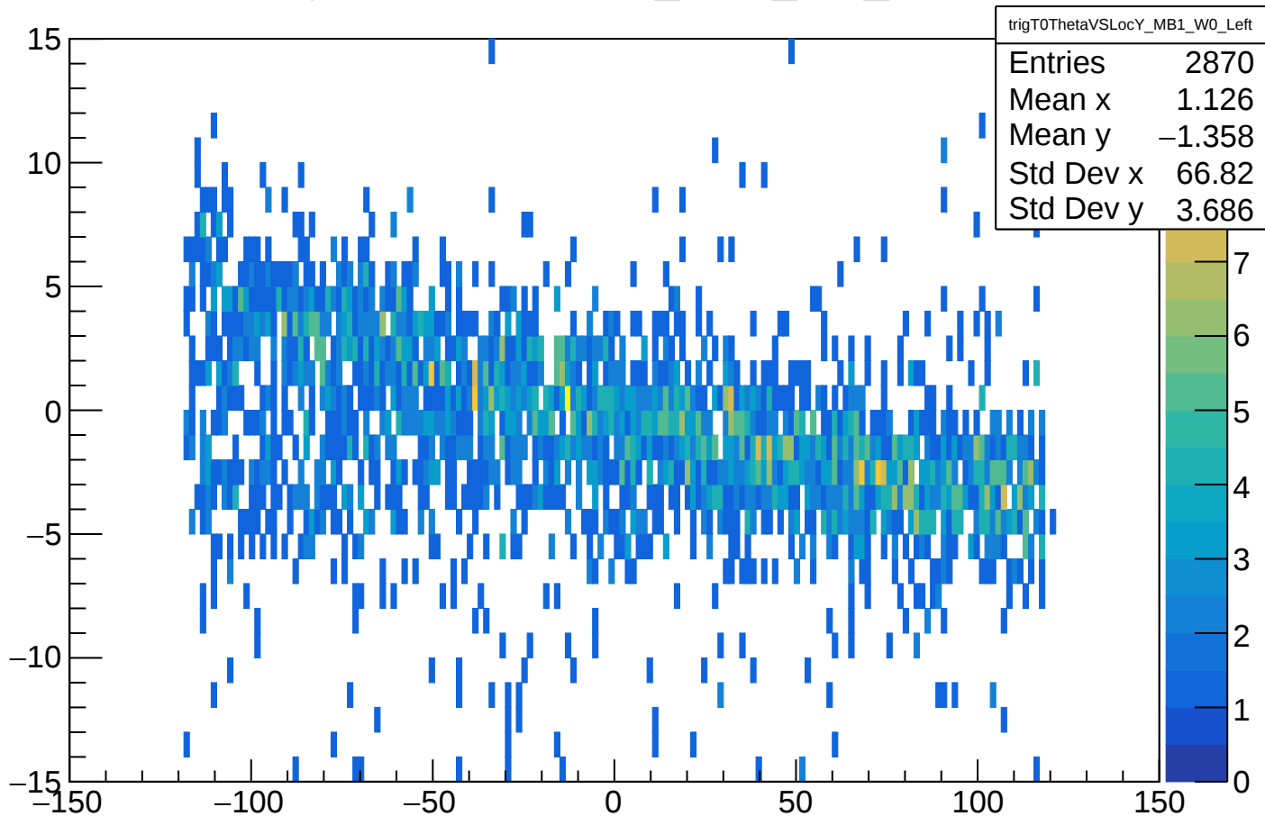
trigT0ThetaVSLocY_MB1_W0_Left
