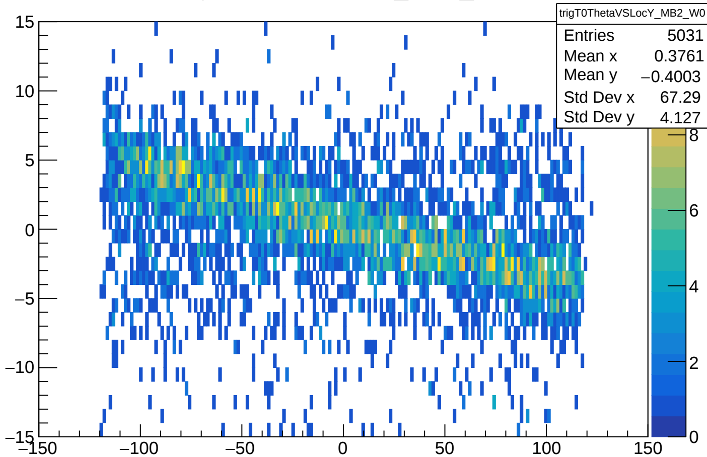
trigT0ThetaVSLocY_MB2_W0
