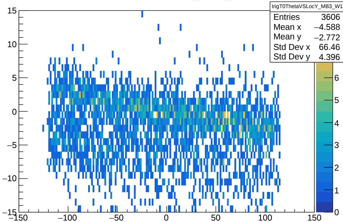
trigT0ThetaVSLocY_MB3_W1
