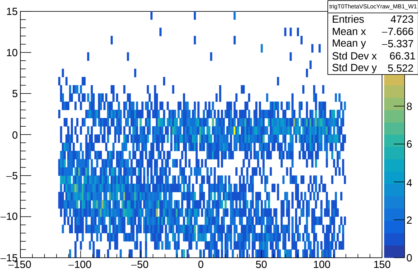
trigT0ThetaVSLocYraw_MB1_W1
