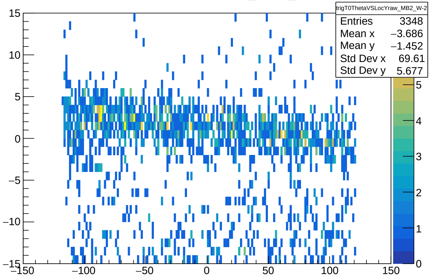
trigT0ThetaVSLocYraw_MB2_W-2
