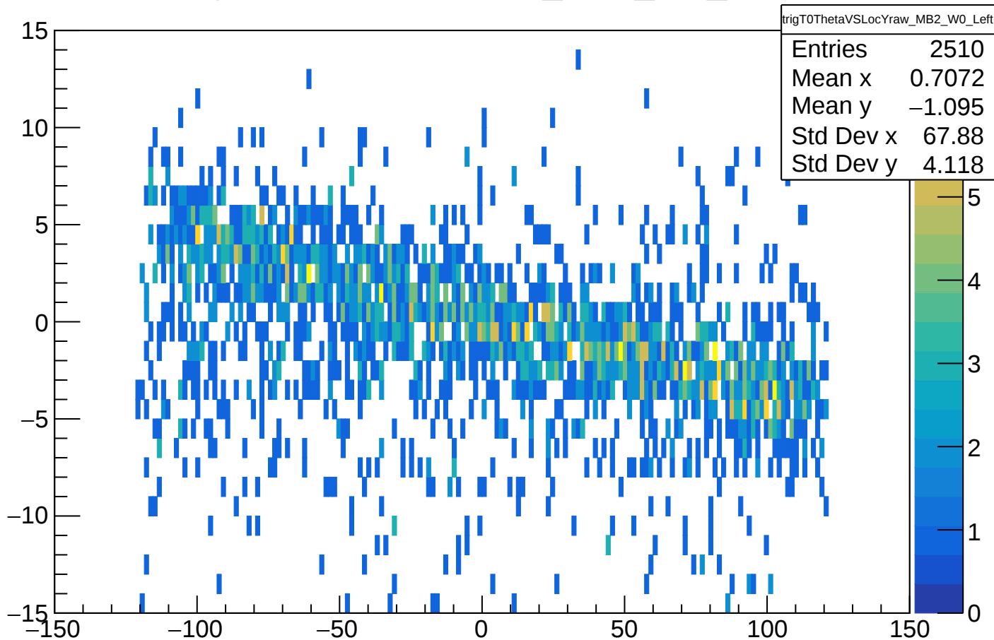
trigT0ThetaVSLocYraw_MB2_W0_Left
