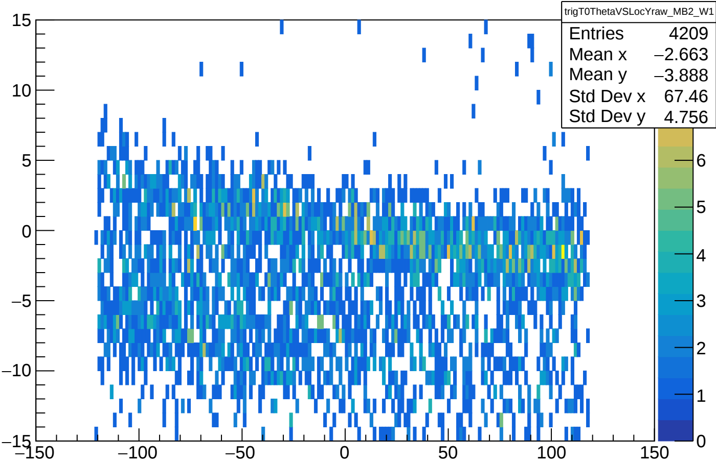
trigT0ThetaVSLocYraw_MB2_W1
