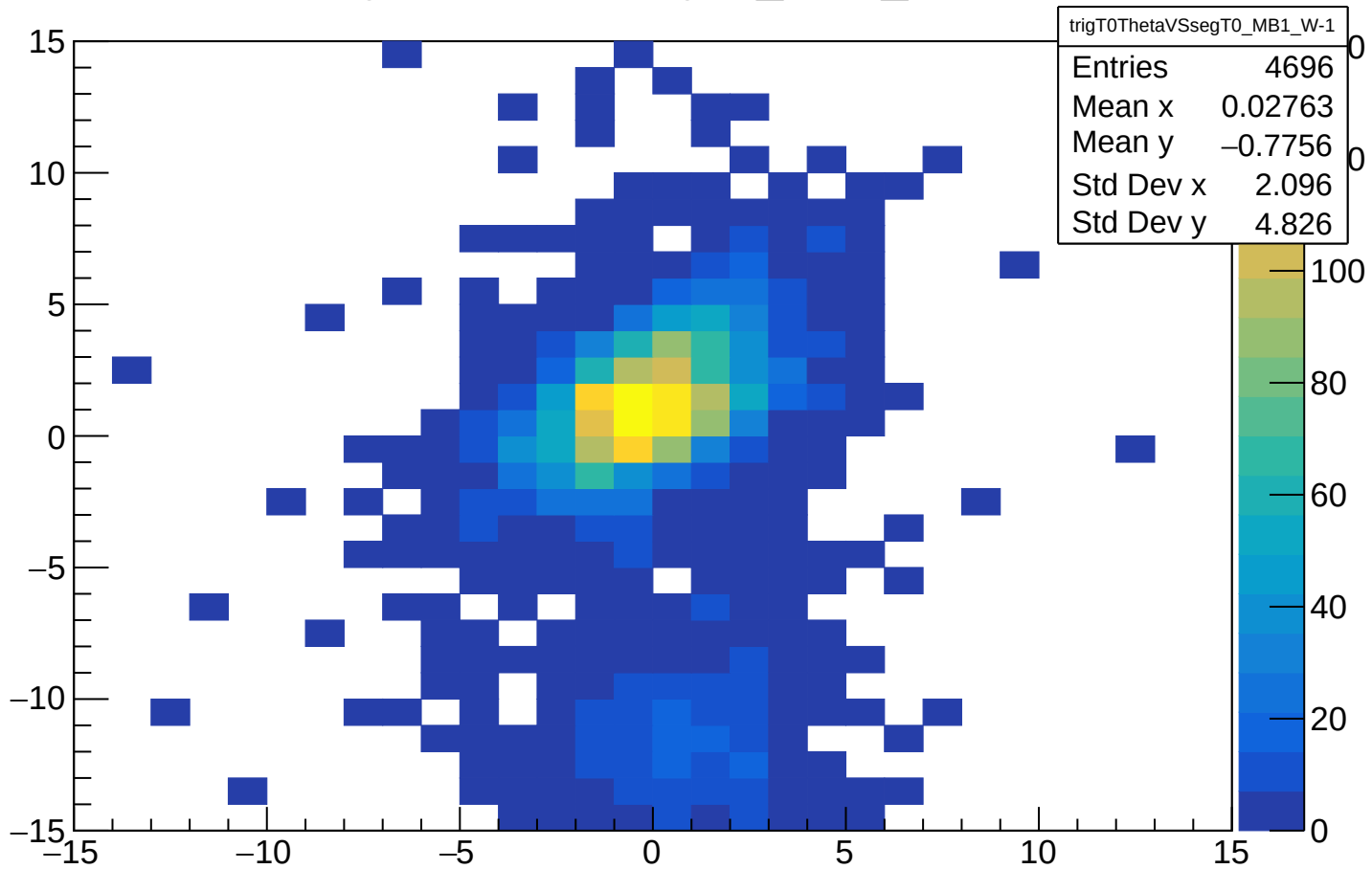
trigT0ThetaVSsegT0_MB1_W-1
