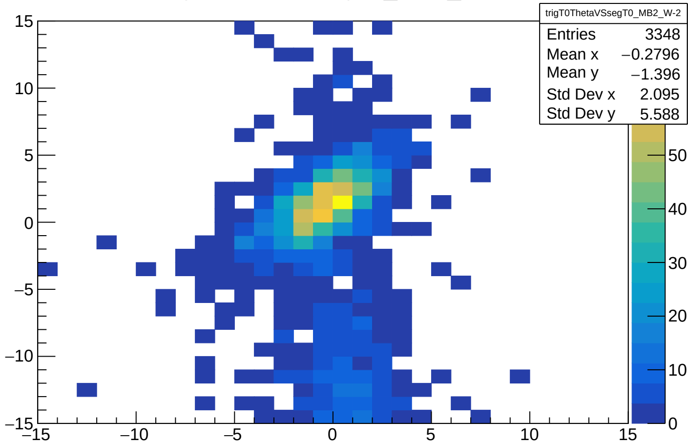
trigT0ThetaVSsegT0_MB2_W-2
