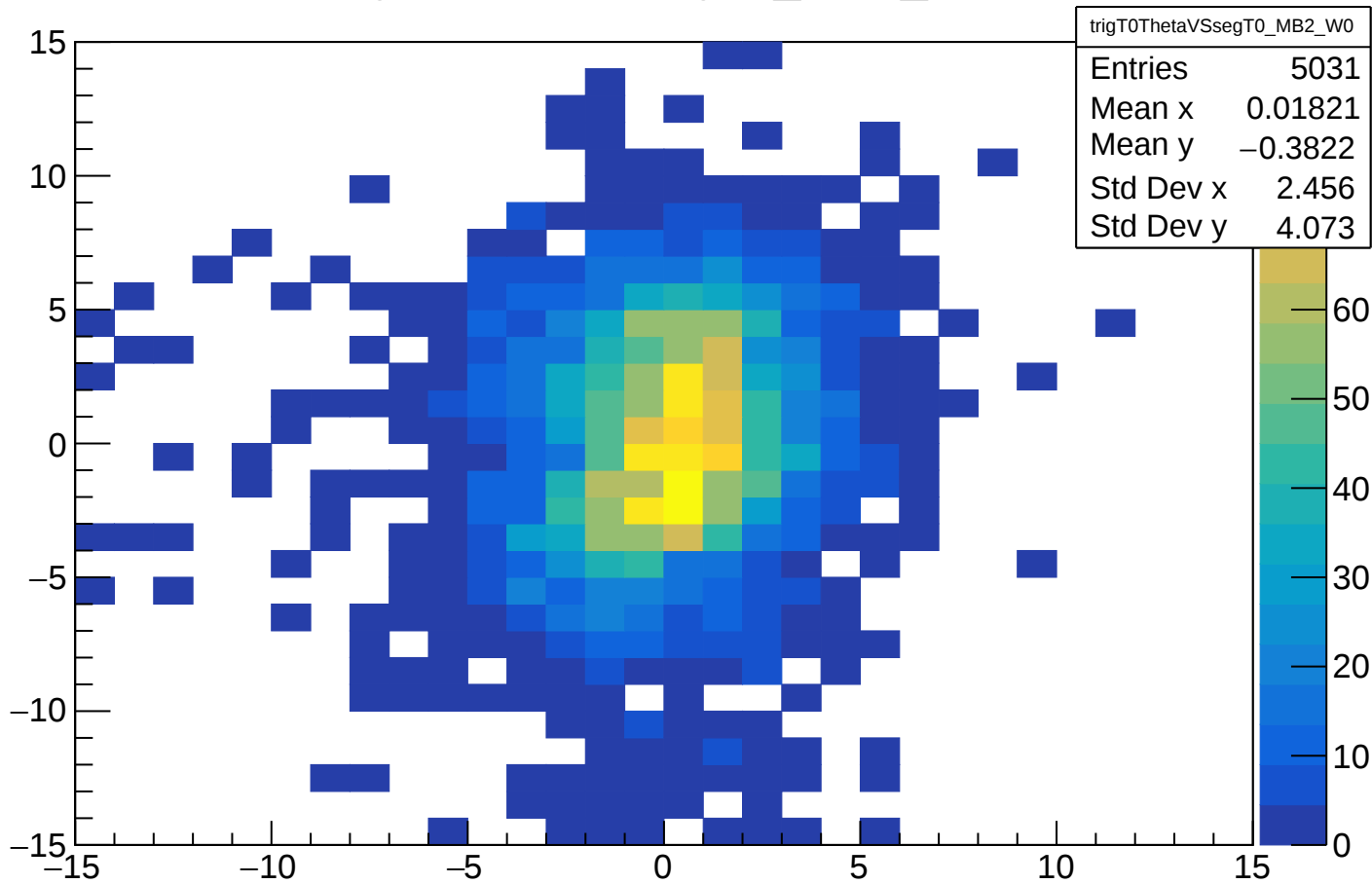
trigT0ThetaVSssegT0_MB2_W0
