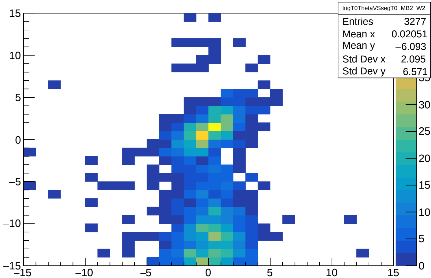
trigT0ThetaVSssegT0_MB2_W2
