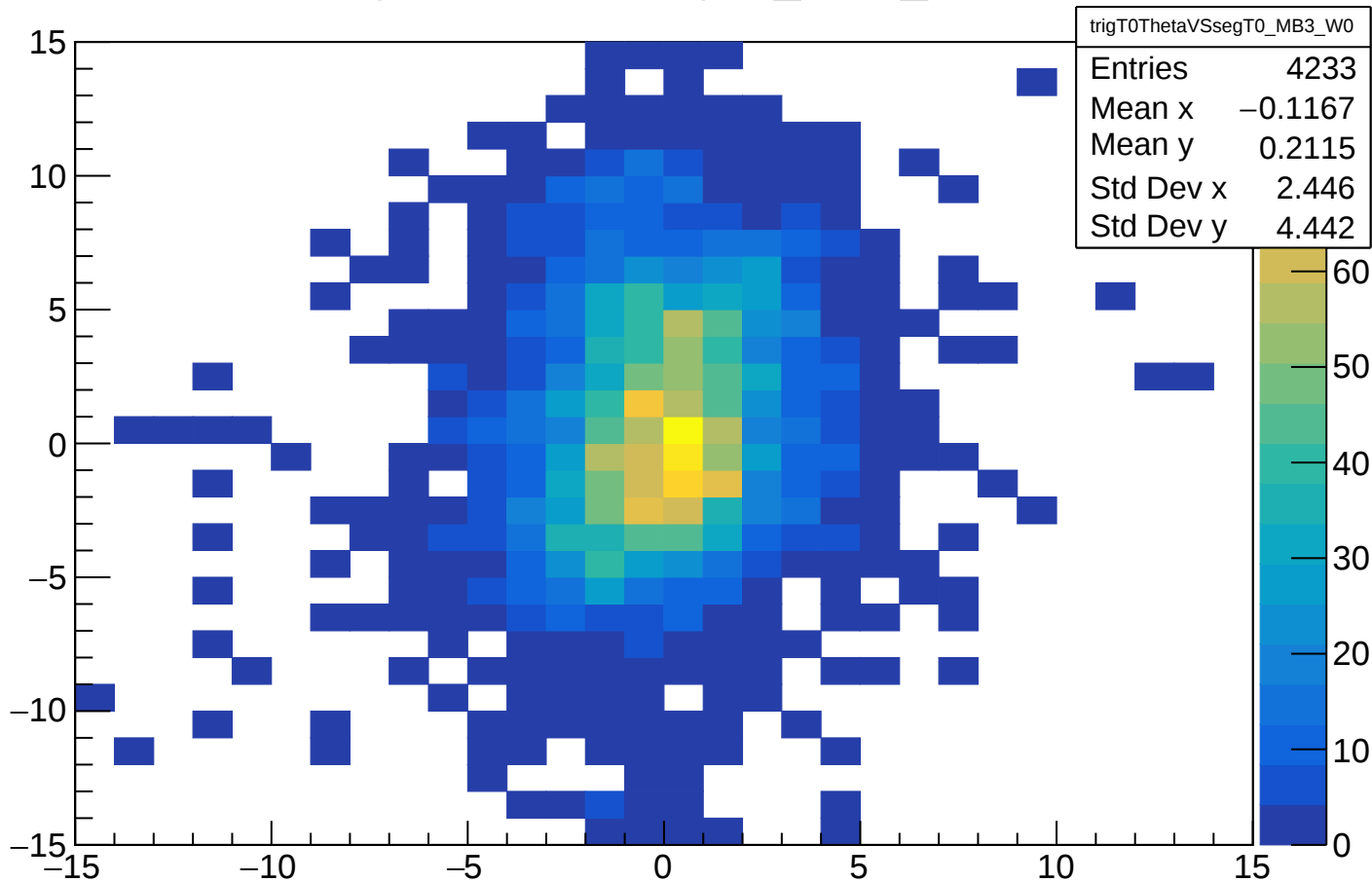
trigT0ThetaVSssegT0_MB3_W0
