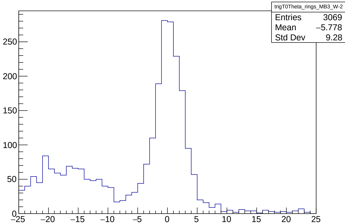
trigT0Theta_rings_MB3_W-2
