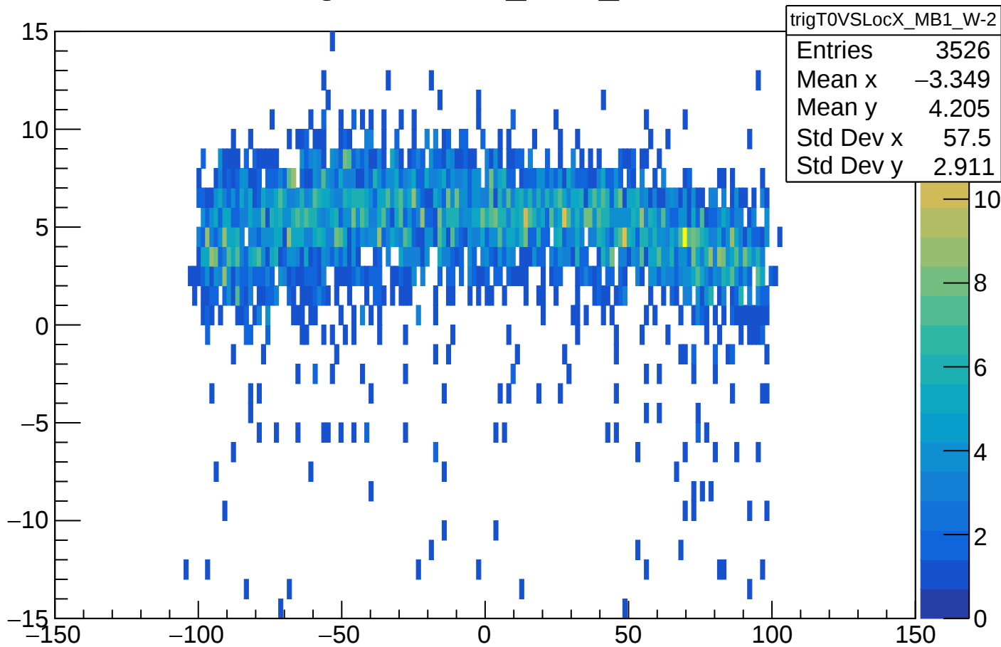
trigT0VSLocX_MB1_W-2
