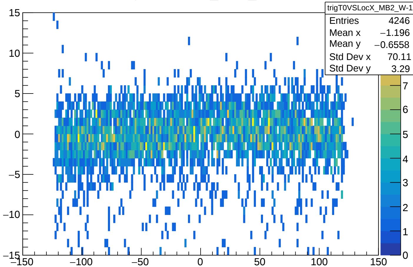
trigT0VSLocX_MB2_W-1
