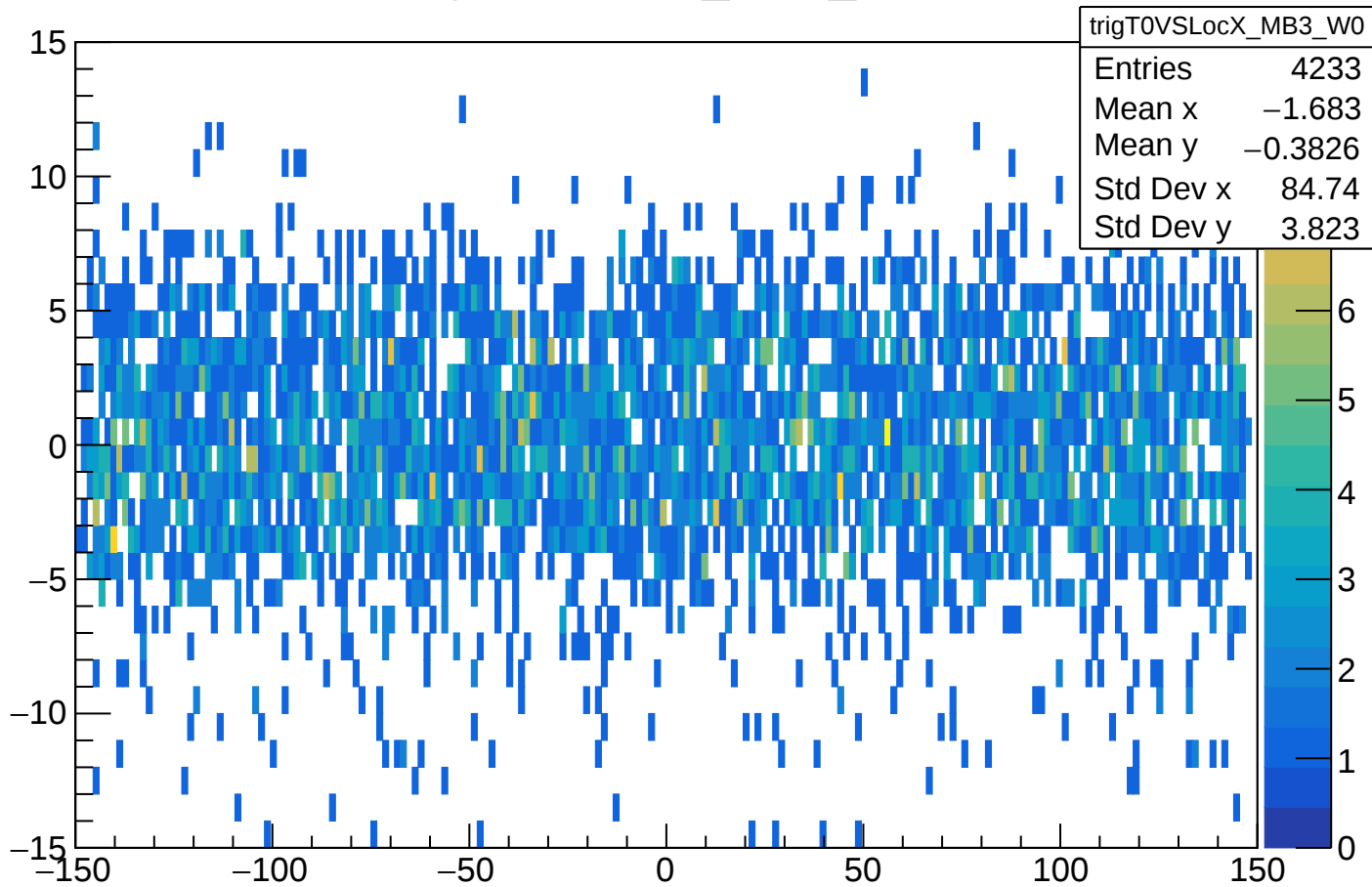
trigT0VSLocX_MB3_W0
