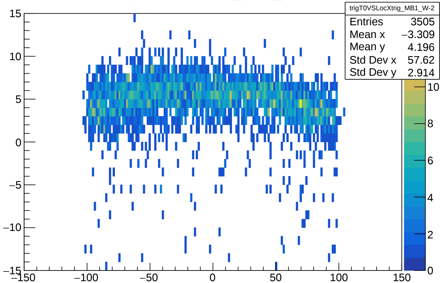
trigT0VSLocXtrig_MB1_W-2
