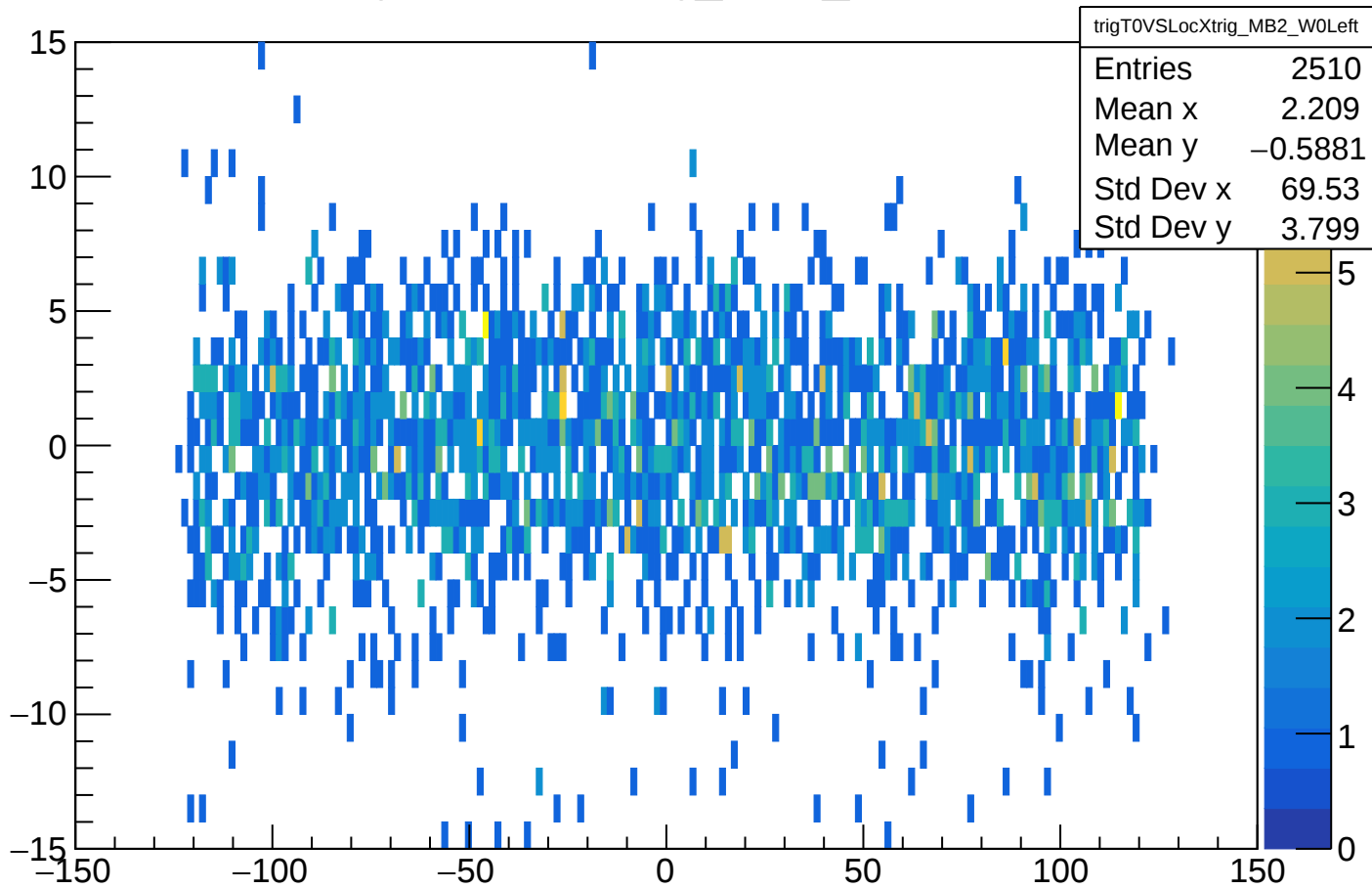
trigT0VSLocXtrig_MB2_W0Left
