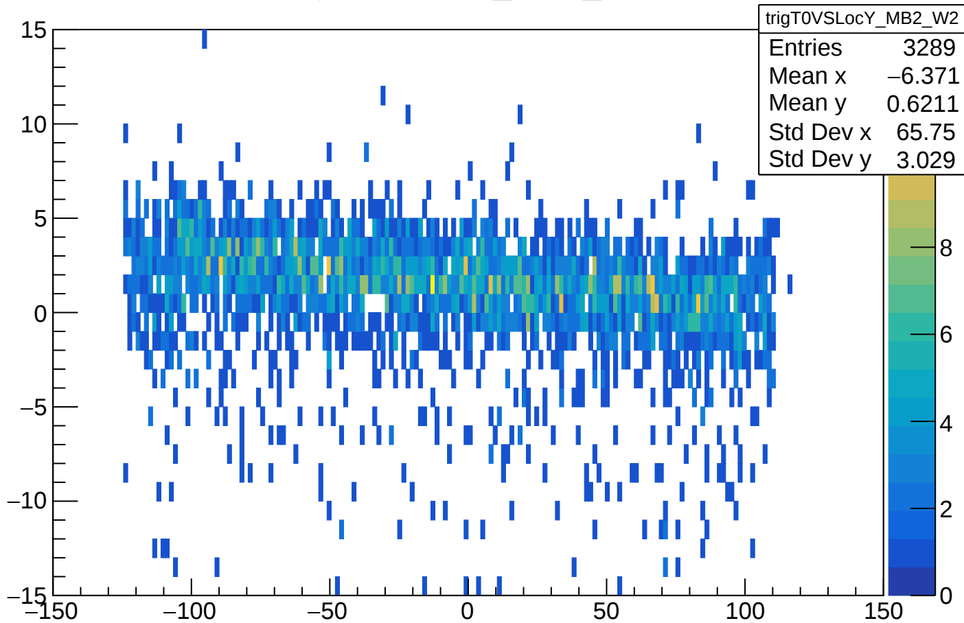
trigT0VSLocY_MB2_W2
