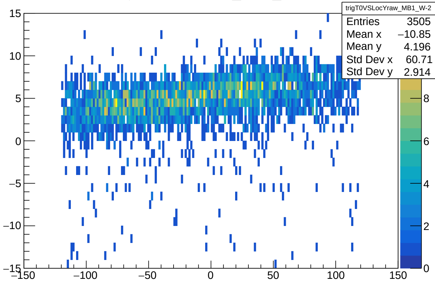
trigTOVSLocYraw_MB1_W-2
