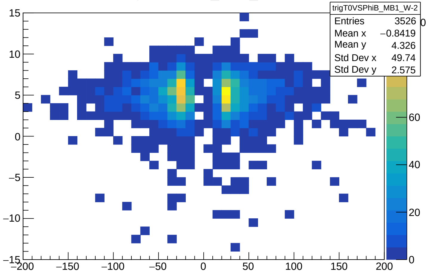
trigT0VSPhiB_MB1_W-2
