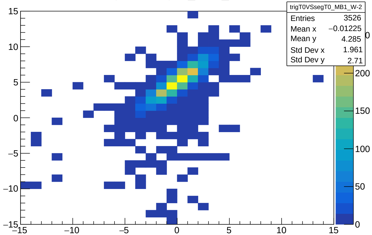
trigT0VSsegT0_MB1_W-2
