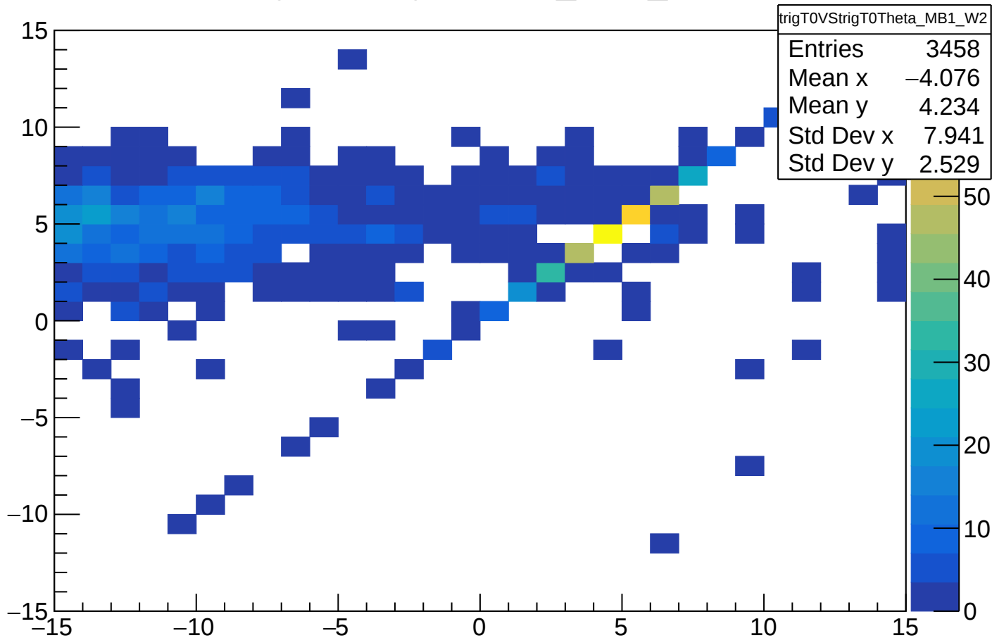
trigT0VStrigT0Theta_MB1_W2
