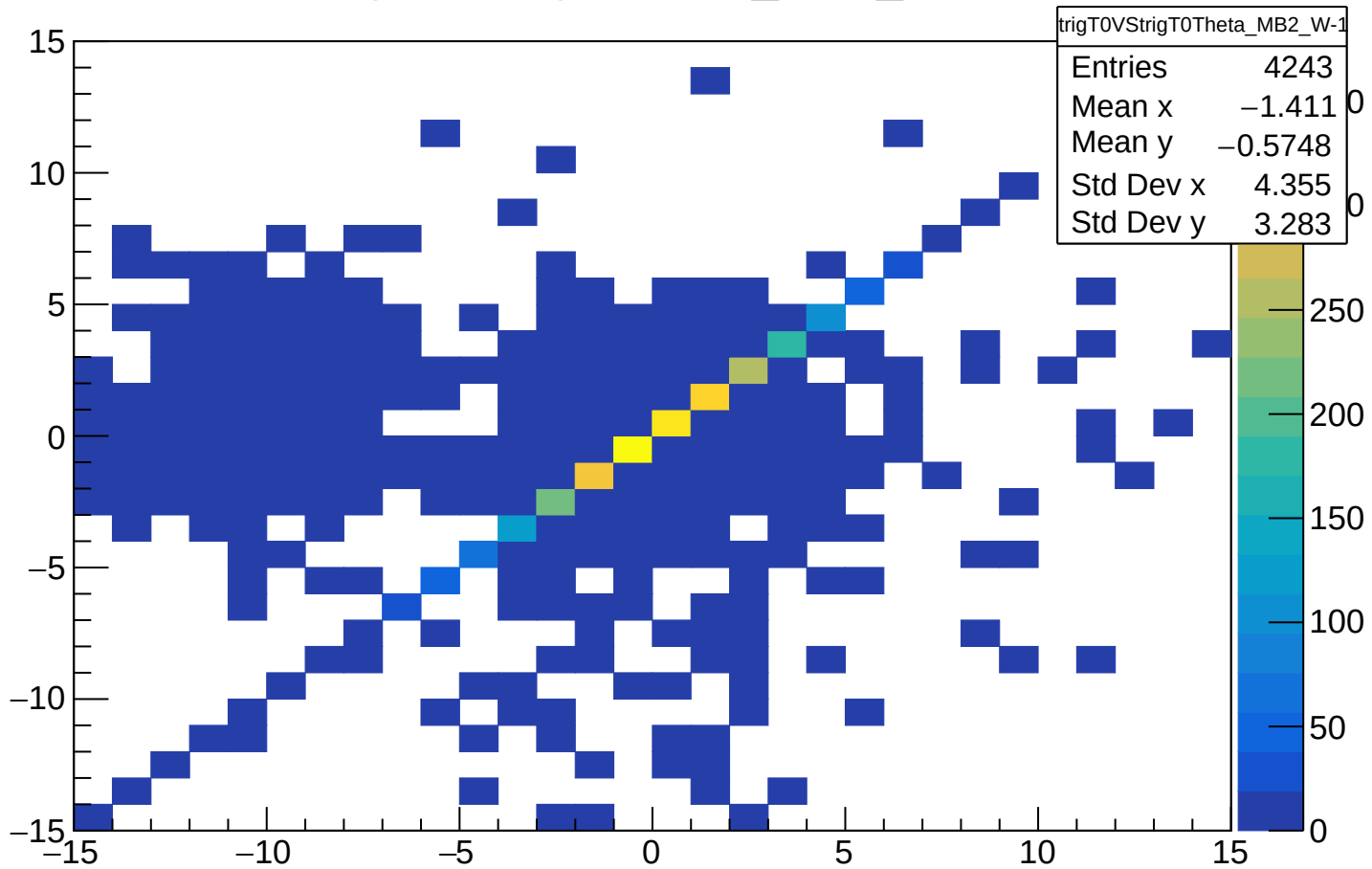
trigT0VStrigT0Theta_MB2_W-1
