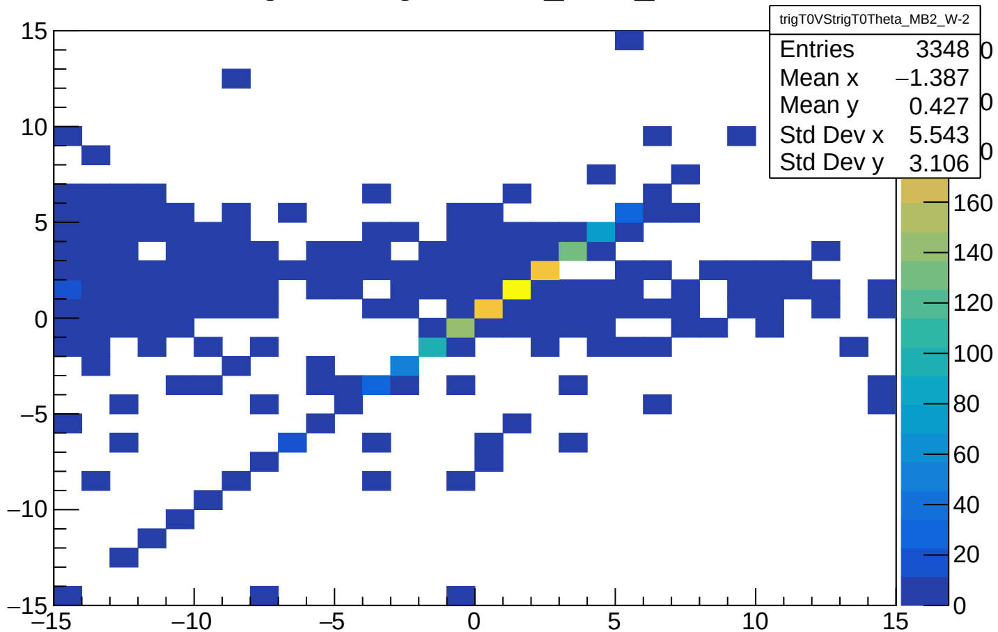
trigT0VStrigT0Theta_MB2_W-2
