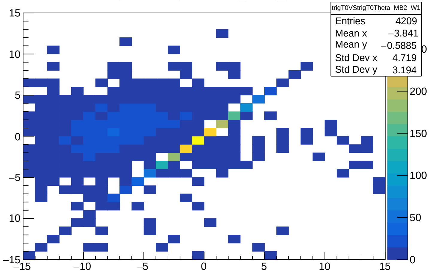
trigT0VStrigT0Theta_MB2_W1
