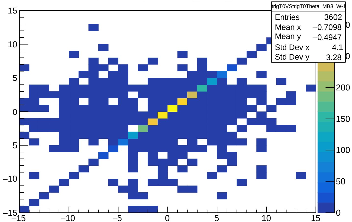
trigT0VStrigT0Theta_MB3_W-1
