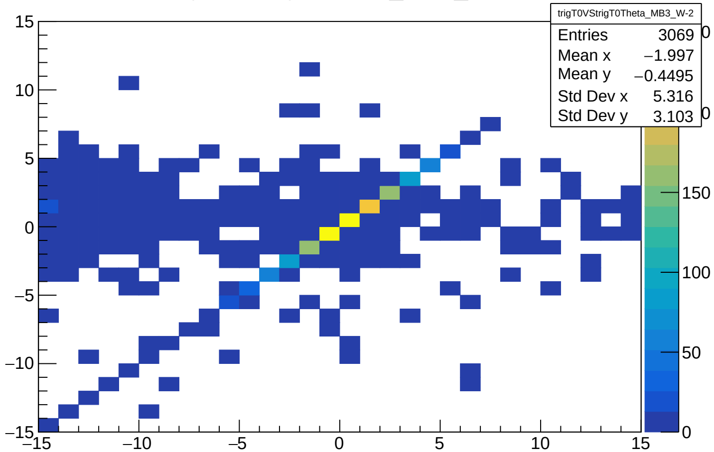
trigTOVStrigT0Theta_MB3_W-2
