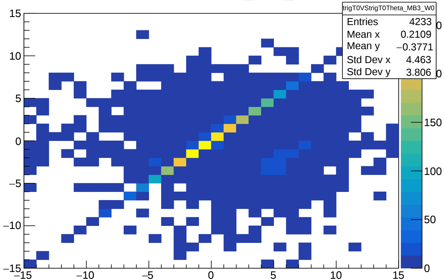
trigT0VStrigT0Theta_MB3_W0
