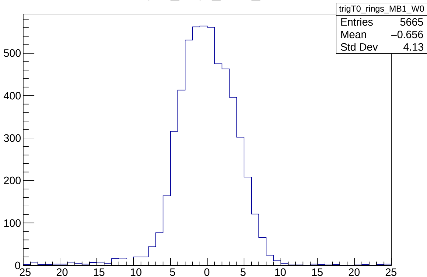
trigT0_rings_MB1_W0
