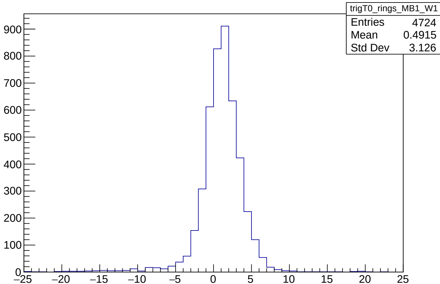
trigT0_rings_MB1_W1
