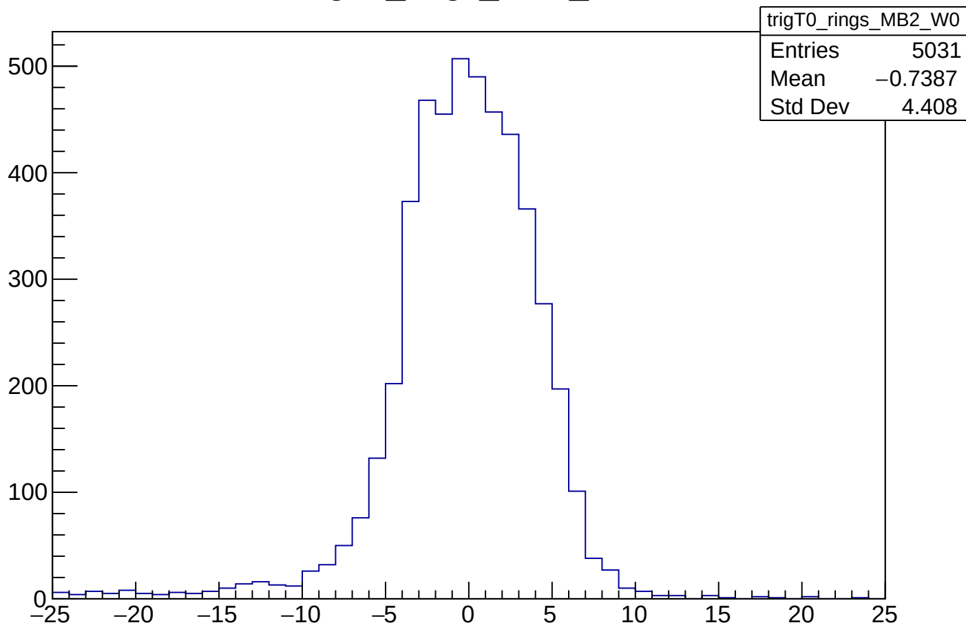
trigT0_rings_MB2_W0
